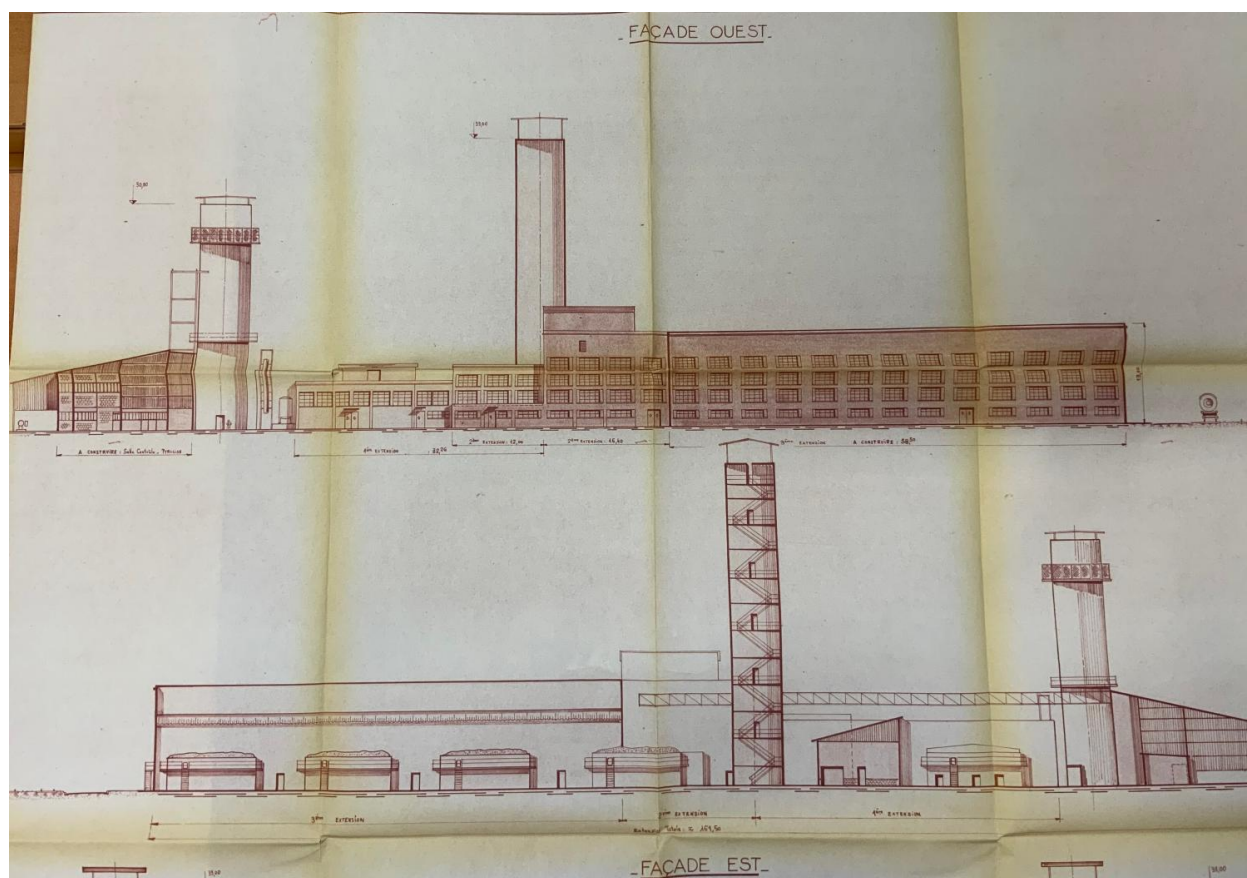
Plan extension façades Est-Ouest, tracé par J. Denis, 1971 (AC Pierre-Bénite : 203 – 45)
