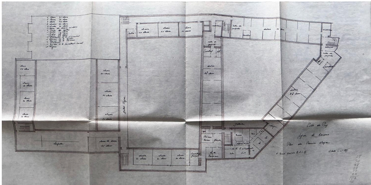
Agrandissement et réorganisation du lycée, avant projet d'E. Grand : plan du 1er étage, mars 1958 (AC Le Puy-en-Velay, 474 W 216)
