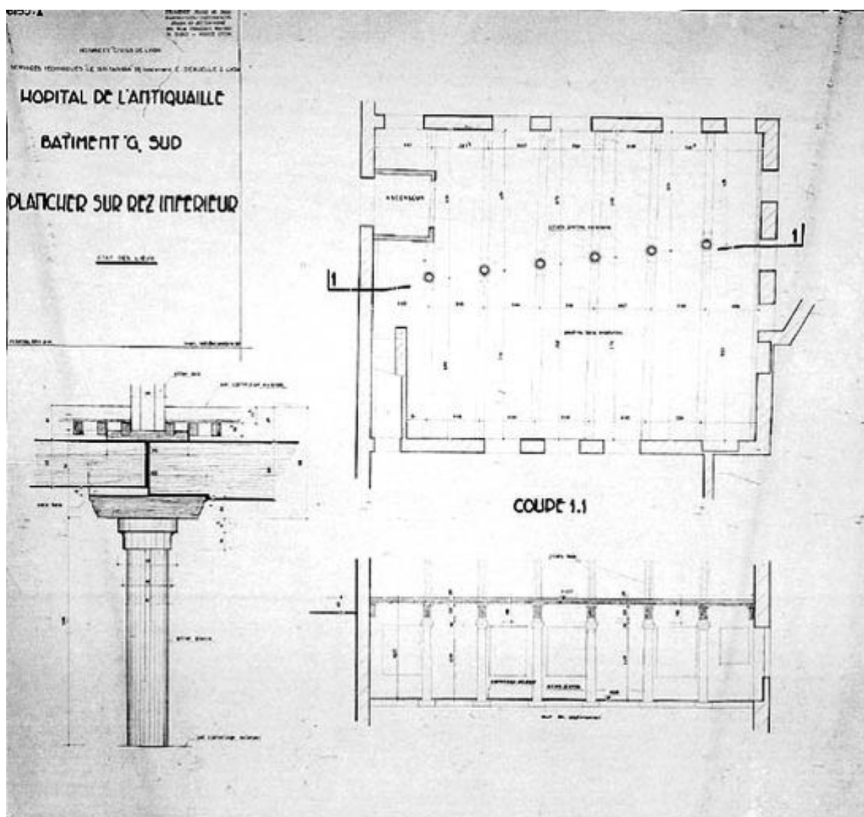
Bâtiment 8, plan et coupe du 2e étage de soubassement, par Raoul et Jean Frairot, 1980
