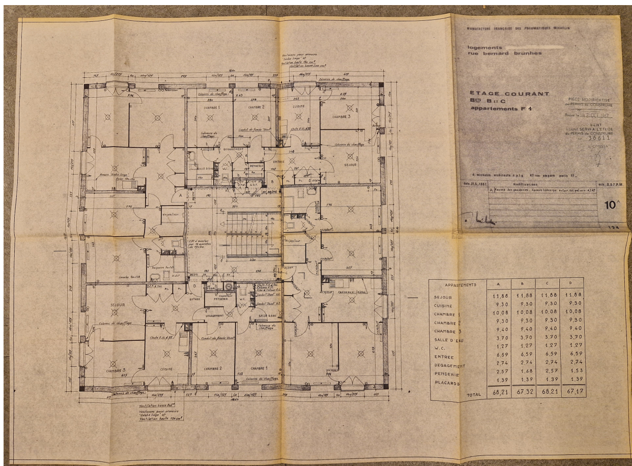
Plan de l'étage courant des bâtiments B et C de la rue Bernard-Brunhes, par Daniel Michelin, 1967.
