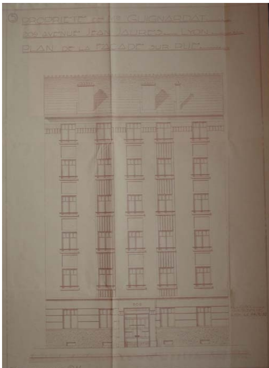
Guignardat ; construction d'un immeuble d'habitation ; façade principale (1935)
