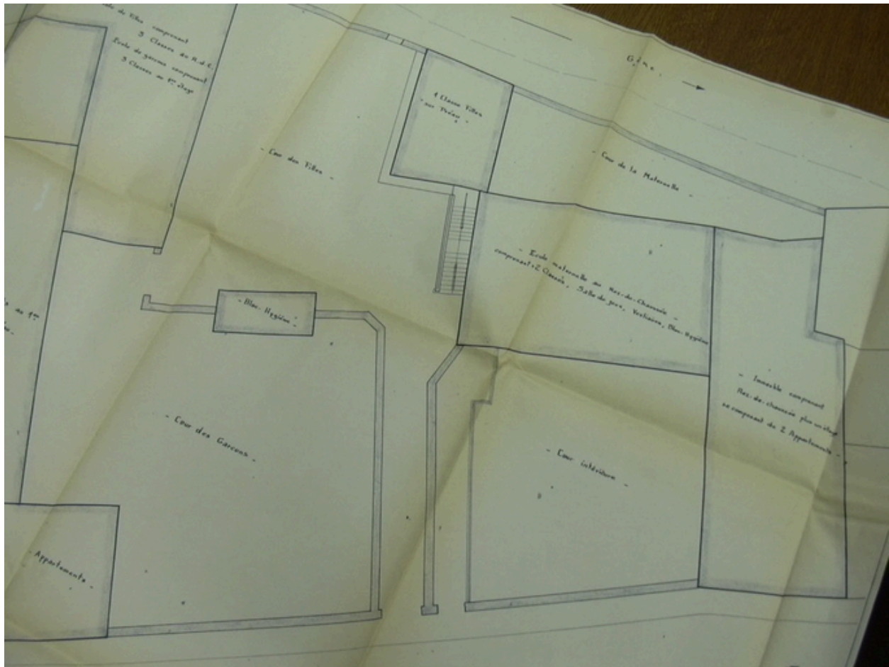
Ecole Lafayette, plan masse, détails
