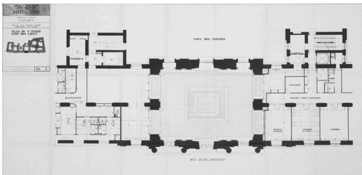
Salle du grand dôme, aménagement des abords, état des lieux. JG Mortamet. [1984-1985 ?] Plan du 1er étage
