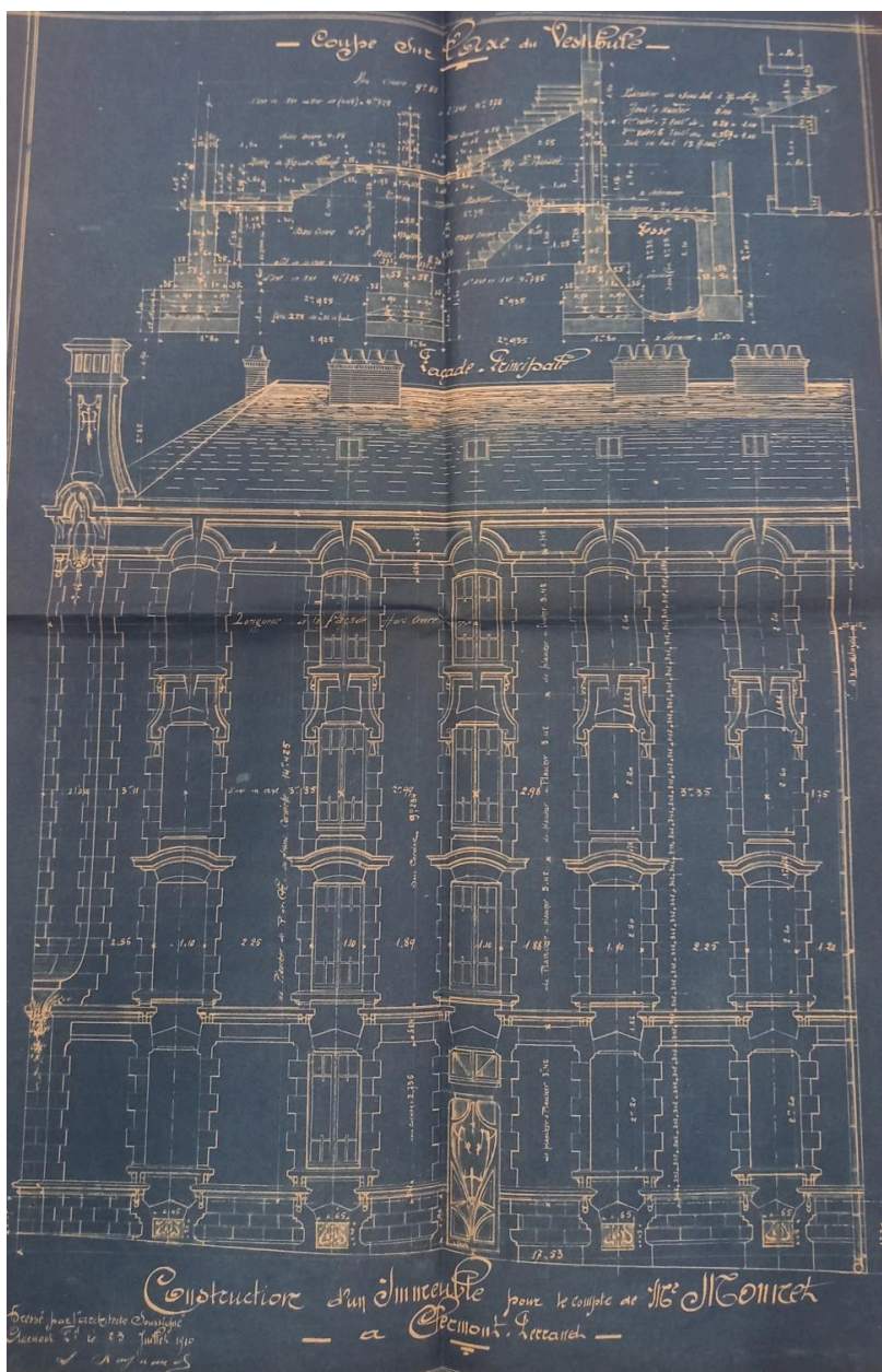
Coupe dans l'axe du vestibule et élévation principale, 1 rue d'Alsace
