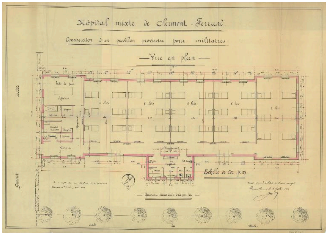
Hôtel-Dieu de Clermont-Ferrand. Le pavillon des militaires, plan du rez-de-chaussée, 8 juillet 1913, Jean Amadon, architecte des hospices.
