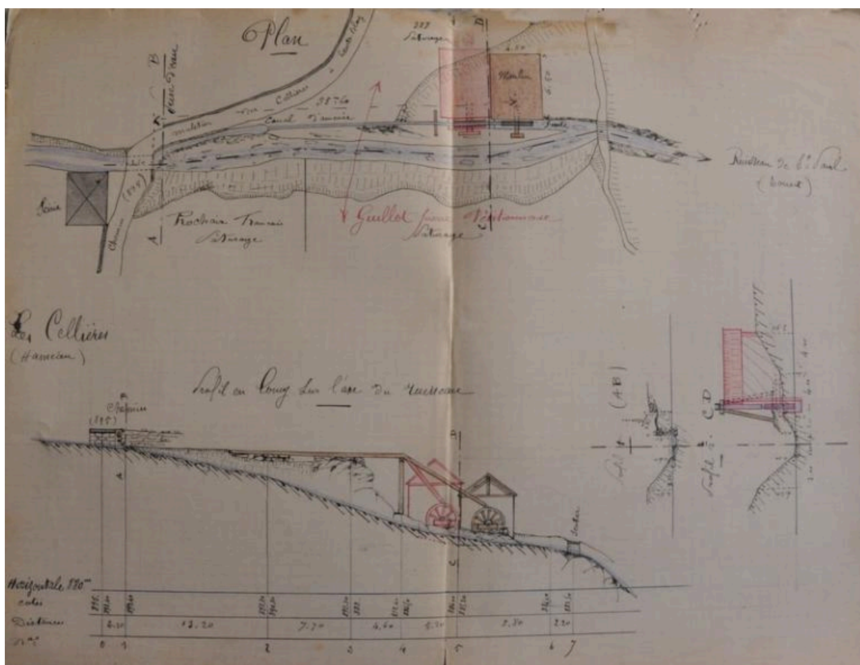
Plan accompagnant la demande de construction de la scierie, 1893 (FR.AD073, 49SPC14).
