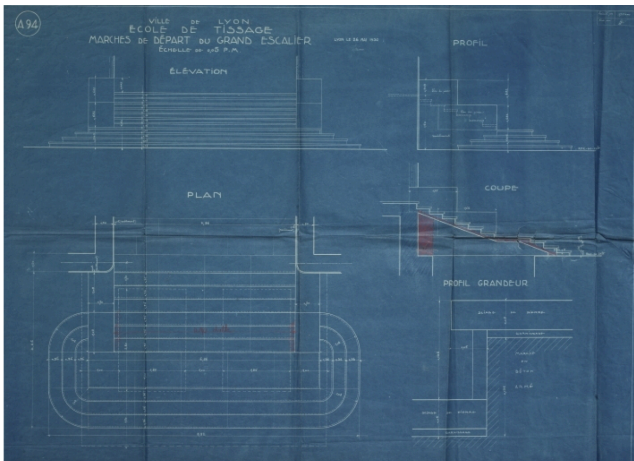
Ecole de tissage, marches de départ du grand escalier, élévation, plan, coupe, profil grandeur, signature illisible, 26 mai 1930. (AC Lyon. 511 WP 002)
