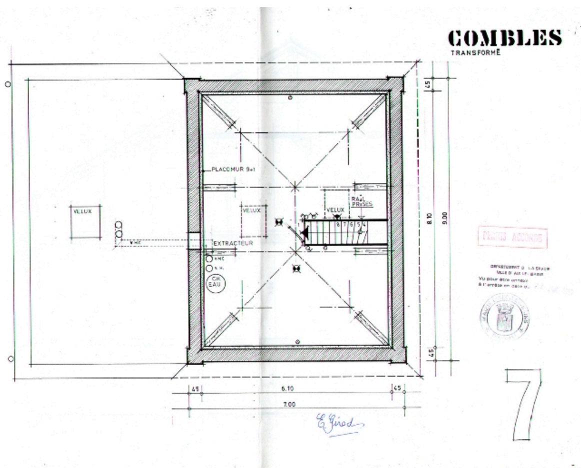
Plan du comble après transformation
