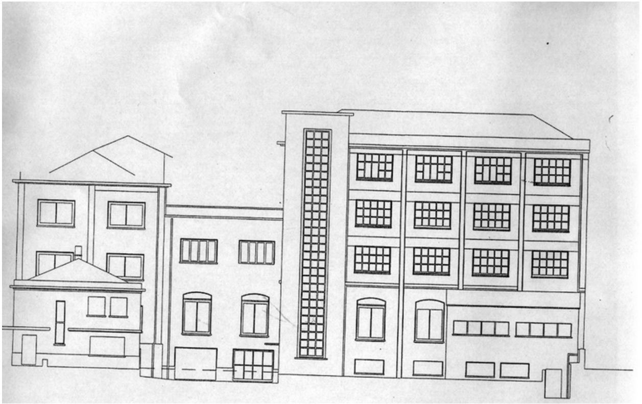
Plan façade est
