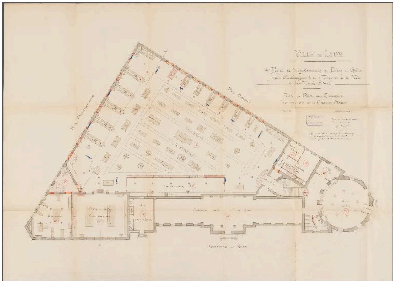
Quatrième projet de transformation du Palais de Glace pour l'aménagement des Muséums de la Ville et du Musée Guimet, plan du rez-de-chaussée au niveau de la grande salle, emplacement des radiateurs, Tony Blein architecte, fond de plan du 25 octobre 1911
