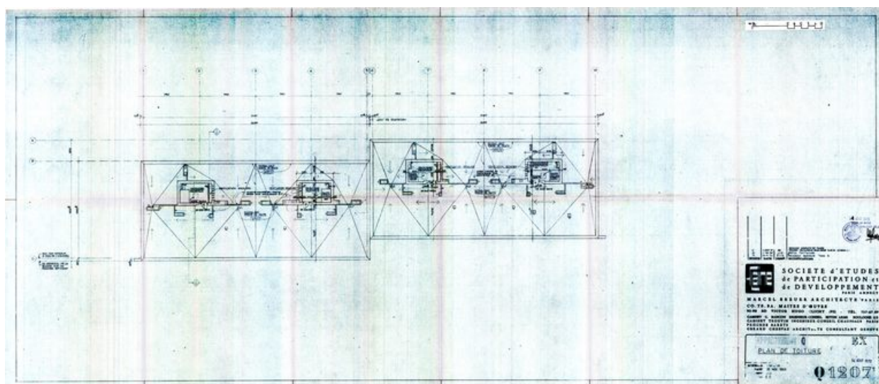
Appartement Q. Plan de toiture. Marcel Breuer architecte, 30 novembre 1969. Modifié les 13 avril, 11 mai et 11 août 1970 (AC Arâches-la Frasse)
