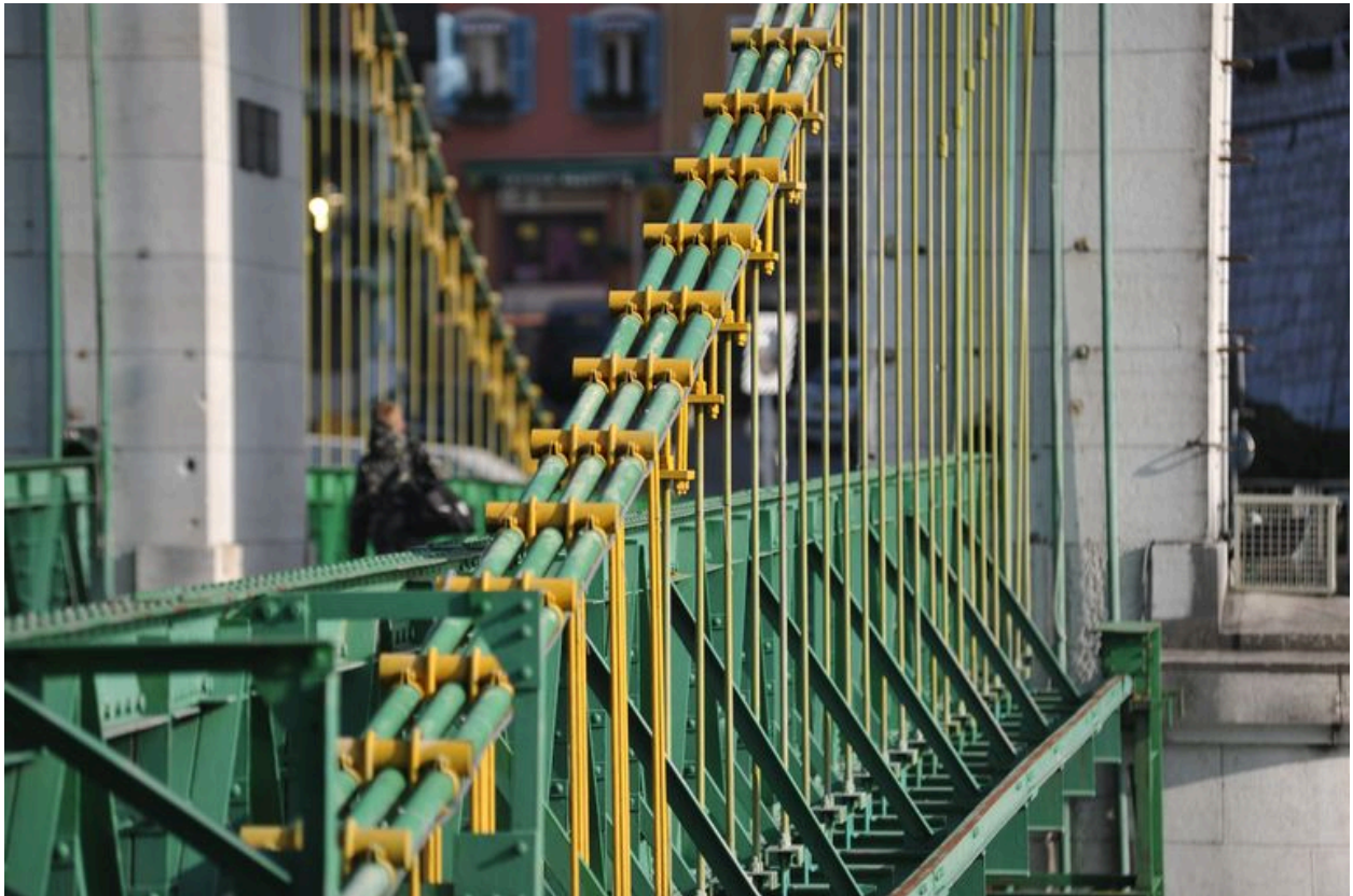
Travée gauche, face aval, vue partielle : câbles porteurs et suspentes (depuis la rive droite)
