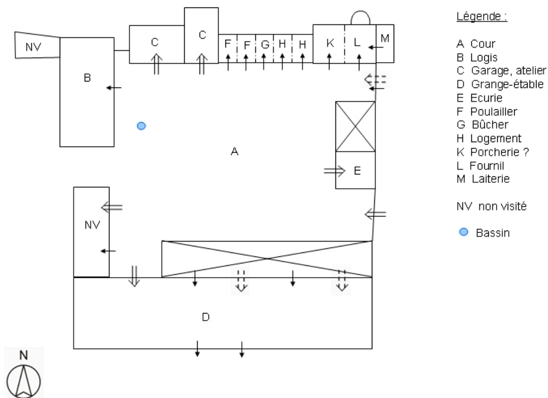
Plan-masse.
