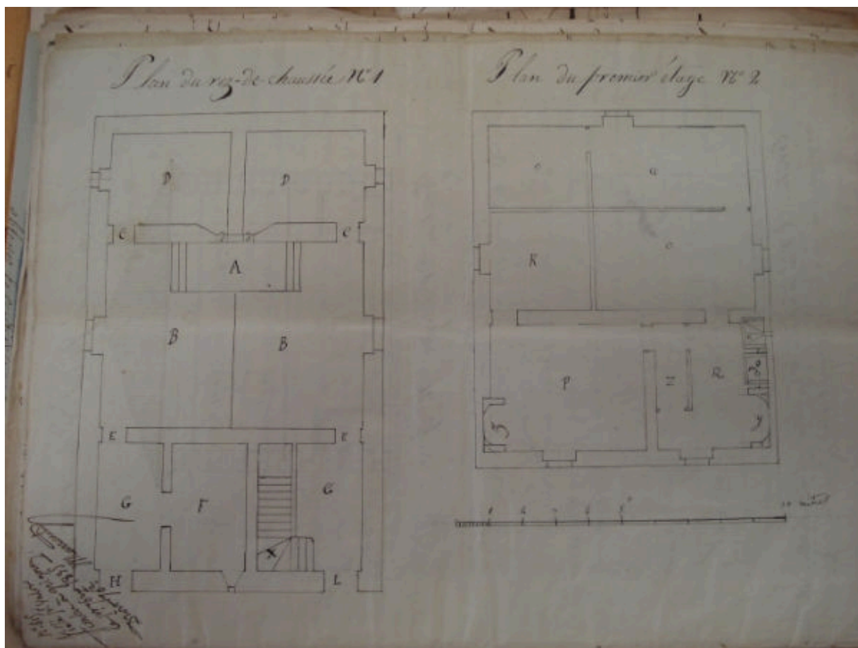
Construction d'une maison d'école avec salle de mairie. Plan du rez-de-chaussée n° 1. Plan du 1er étage n° 2.
