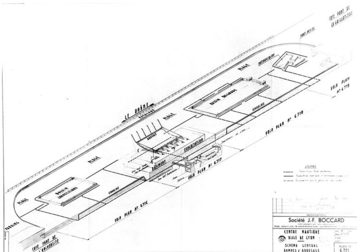
Vue axonométrique de la piscine depuis l'est / Soc. J.-F. Boccard, 4 octobre 1962 (Arch. mun. Lyon. 0002 S 00946)
