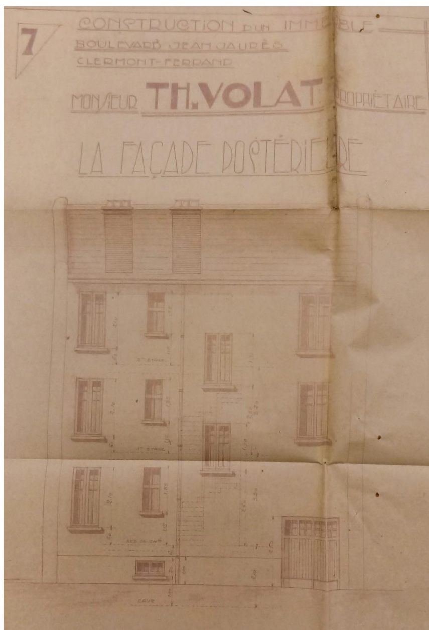
Elévation postérieure
