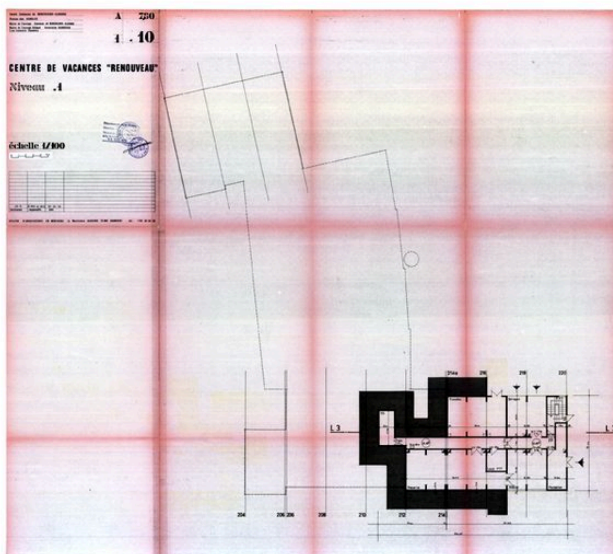
Plan du niveau -1 / Atelier d'Architecture en Montagne, Guy Rey-Millet, Jean-Gustave Orth, 18 janvier 1973 (AC Montricher-Albanne)
