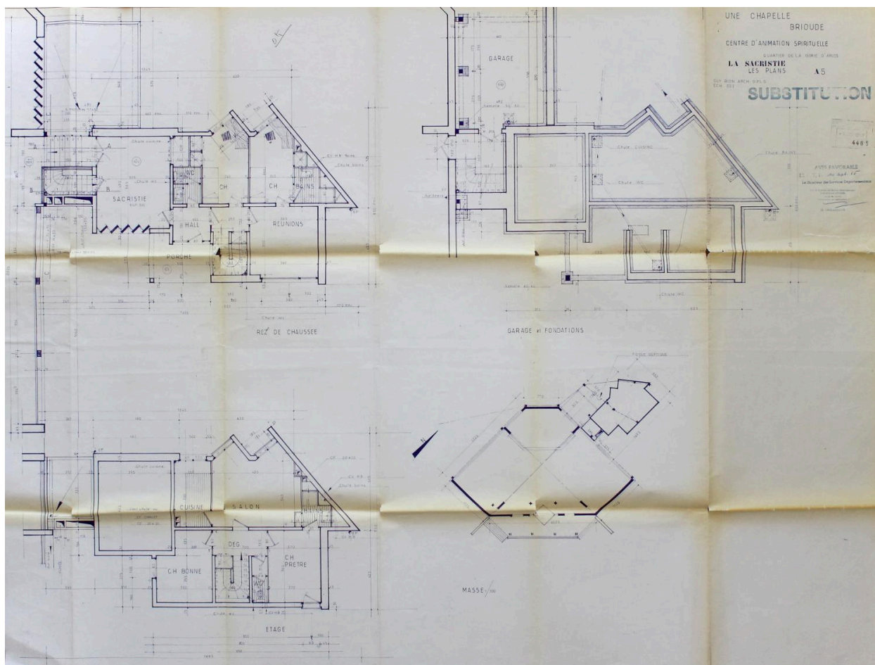
Brioude, chapelle de la Borie Darles, plan d'implantation et plans des niveaux de la sacristie et du logement (seconde version non définitive, non datée, vers juin 1965), Guy Bion architecte, Archives de la paroisse Saint-Julien de Brioude.
