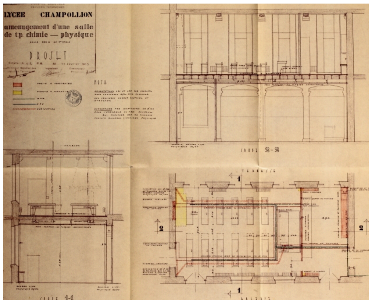
Aménagement d'une salle de TP Chimie-Physique, 1963. Document figuré. Plan. Archives municipales, Grenoble. 4 M 70
