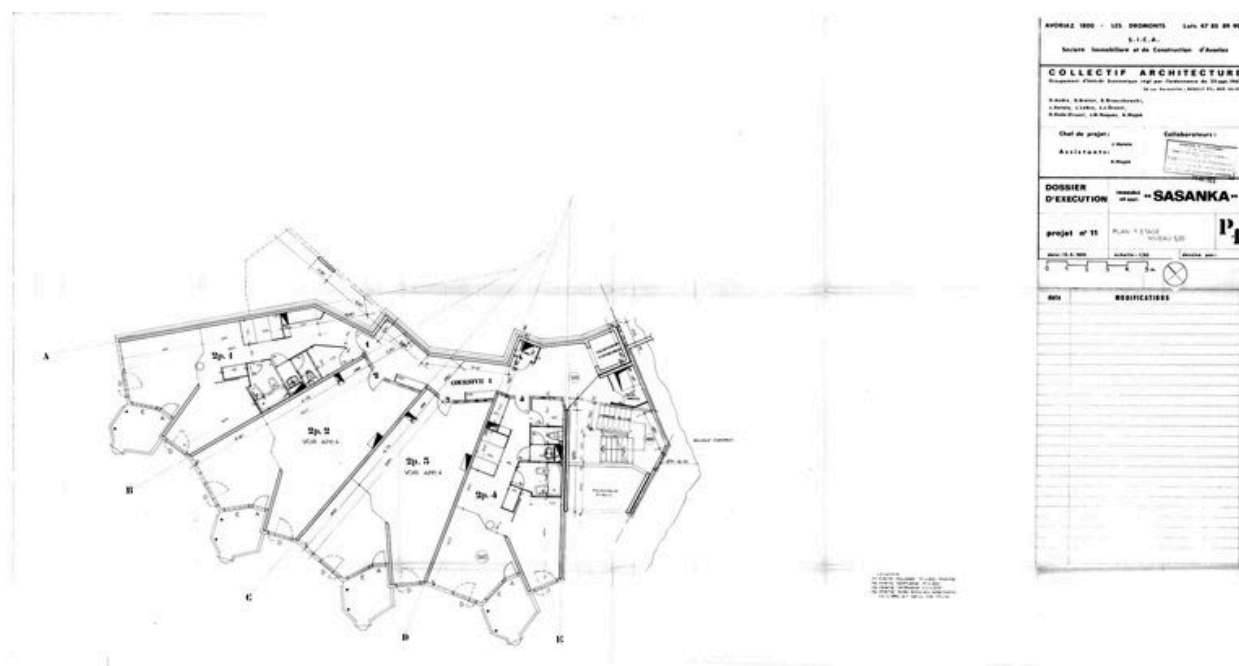
Dossier d'exécution / Collectif Architecture, 15 juin 1969. Plan du 1er étage (AC Morzine)
