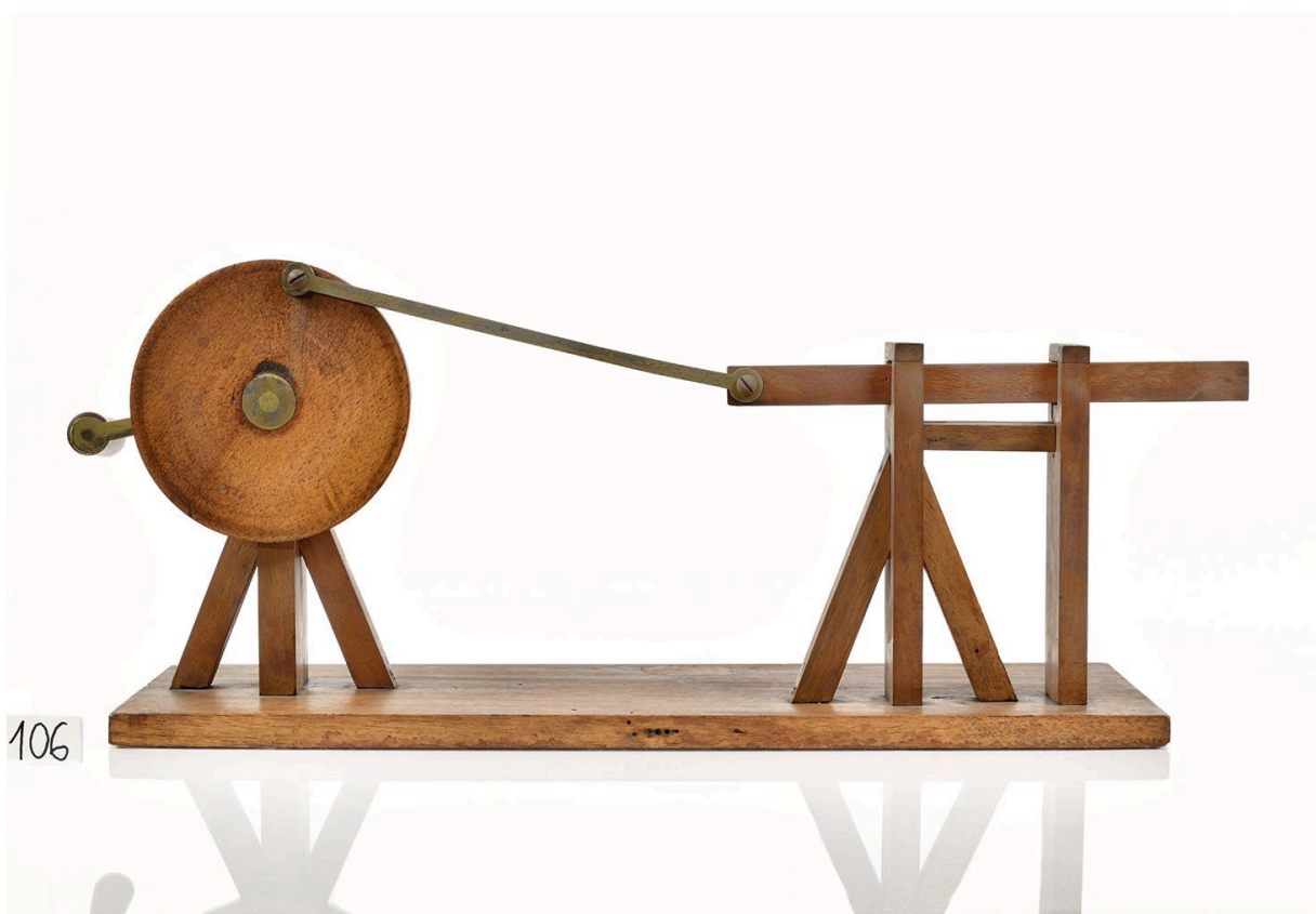
Mouvement circulaire continu changé en rectiligne alternatif, exemplaire 1, vue 2
