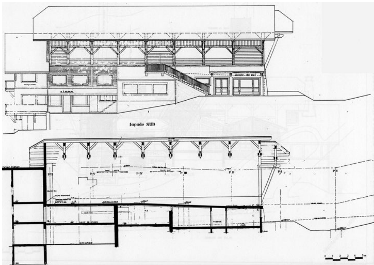
Gare inférieure. Elévation sud et coupe longitudinale / [Pierre Duclos, 1985]
