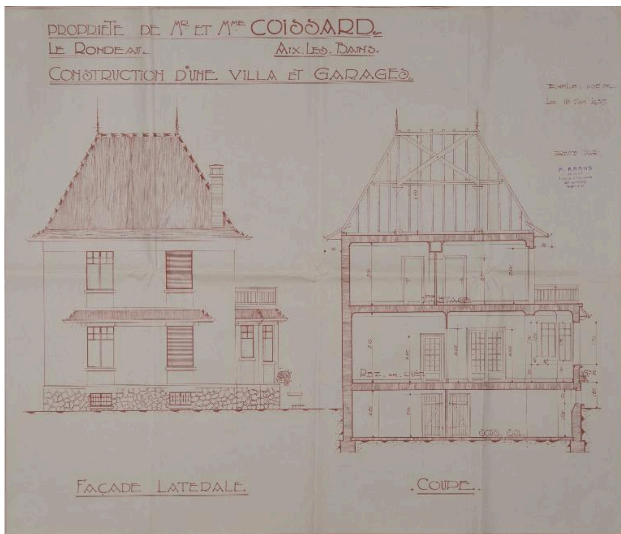
Elévation latérale et coupe transversale
