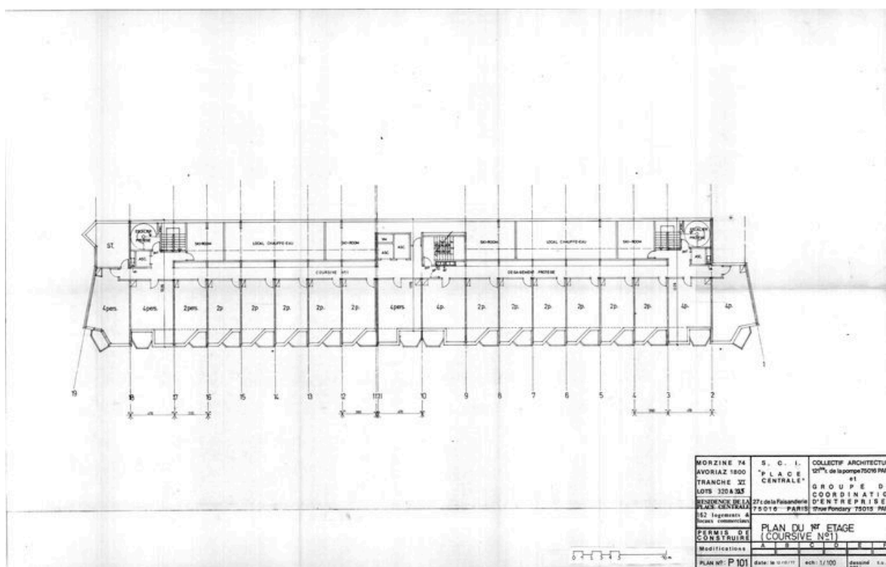
Plan du 1er étage (coursive n° 1) / Collectif architecture et groupe de coordination d'entreprise, 12 octobre 1977 (AC Morzine)
