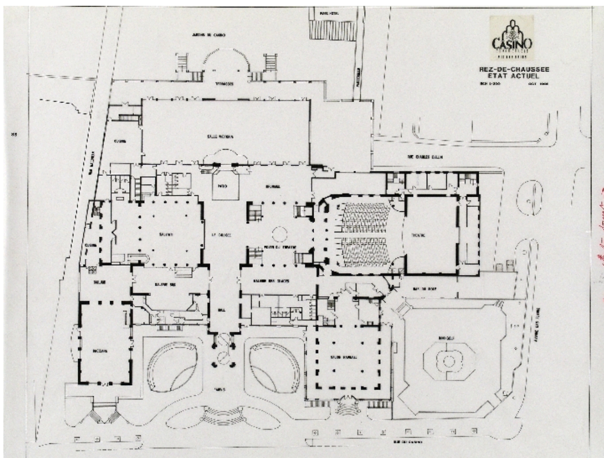
Plan du rez-de-chaussée de l'ensemble théâtre et casino
