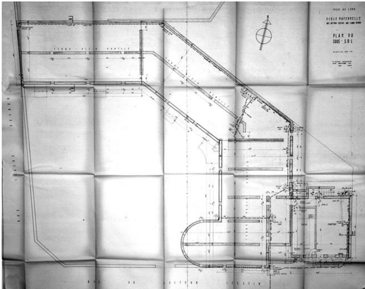
Plan du sous-sol, R. Fauvet architecte. 1:50, mai 1965
