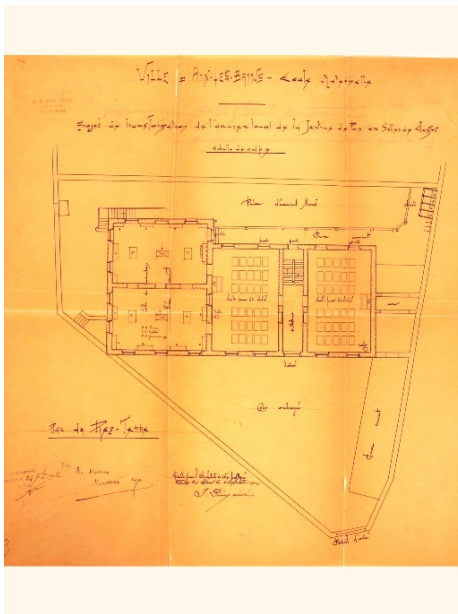
Plan du rez-de-chaussée, 1902
