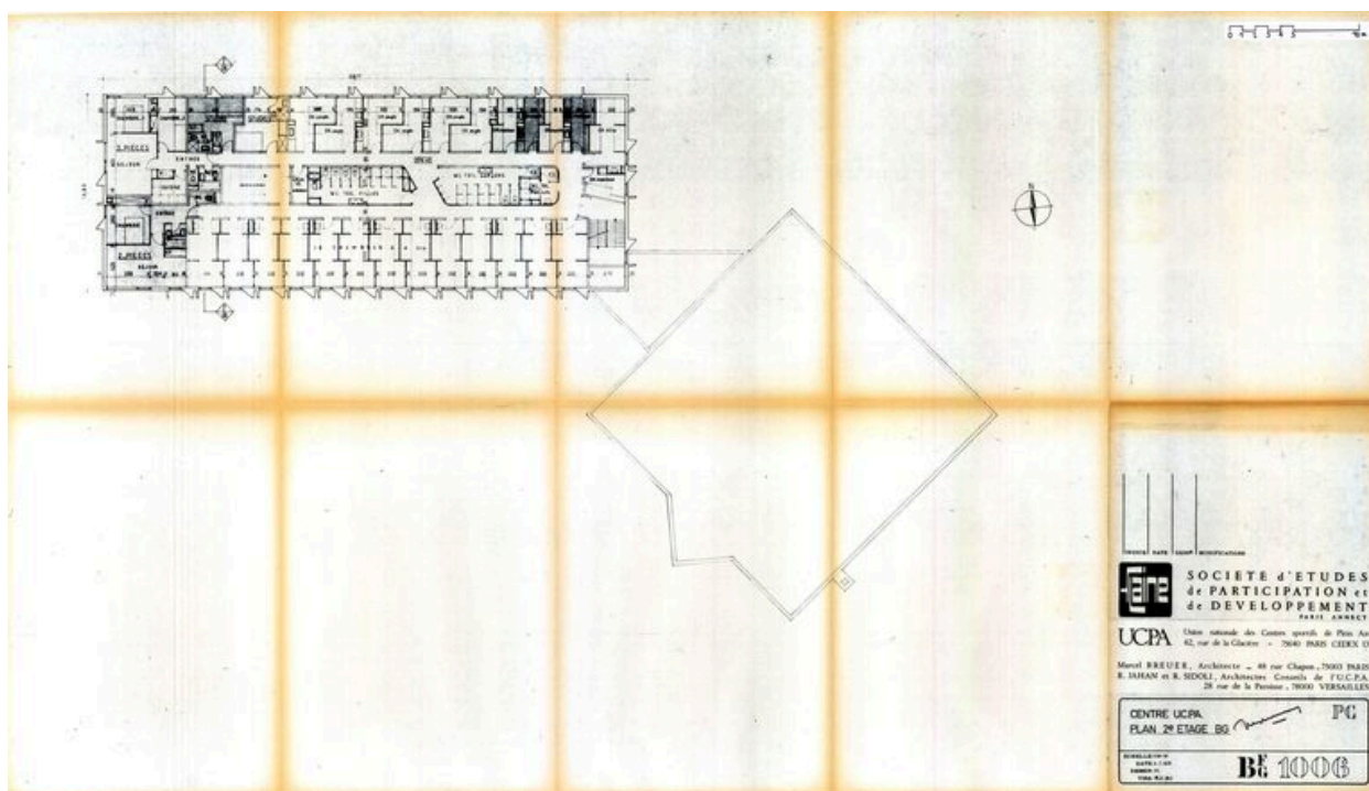
Plan 2e étage BG. Marcel Breuer architecte, R. Jahan et R. Sadoli architectes conseils de l'UCPA, 9 juillet 1975 (AC Magland)
