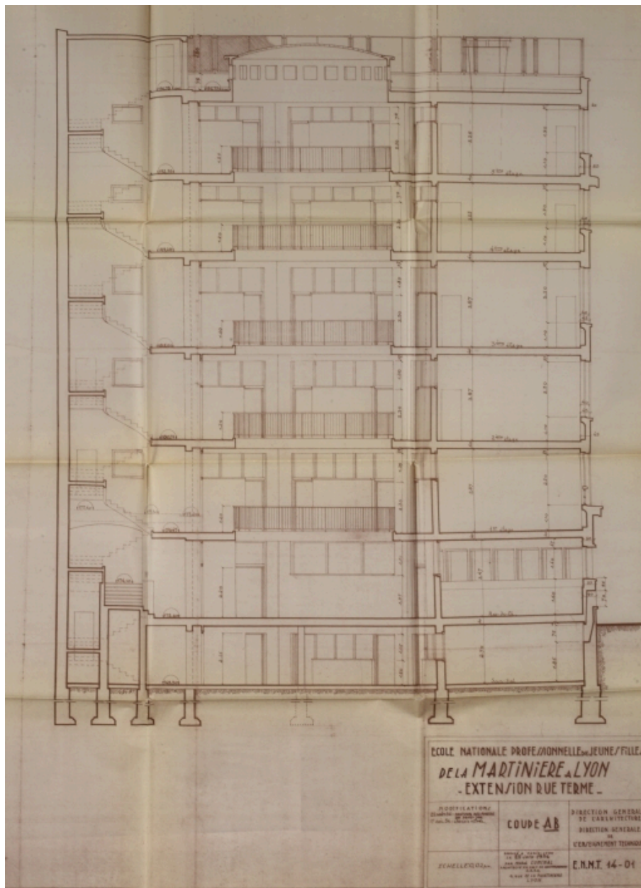
E.N.M.T. 14-01 Coupe AB. Modifications du 25 août 1956. Document figuré. Coupe. Archives du Lycée de la Martinière (intendance Augustins). non coté
