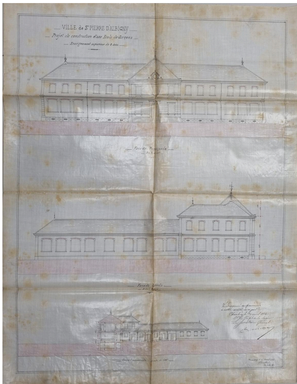
Ville de Saint-Pierre-d'Albigny. Projet de construction d'une école de garçons. Enseignement supérieur de 2 ans [3] Façade principale. Echelle de 0,01. Façade latérale. Echelle de 0,01. Coupe transversale. Echelle de 0,005. Charles Coustard (architecte), 1883 (AD Savoie. 2O 2695).
