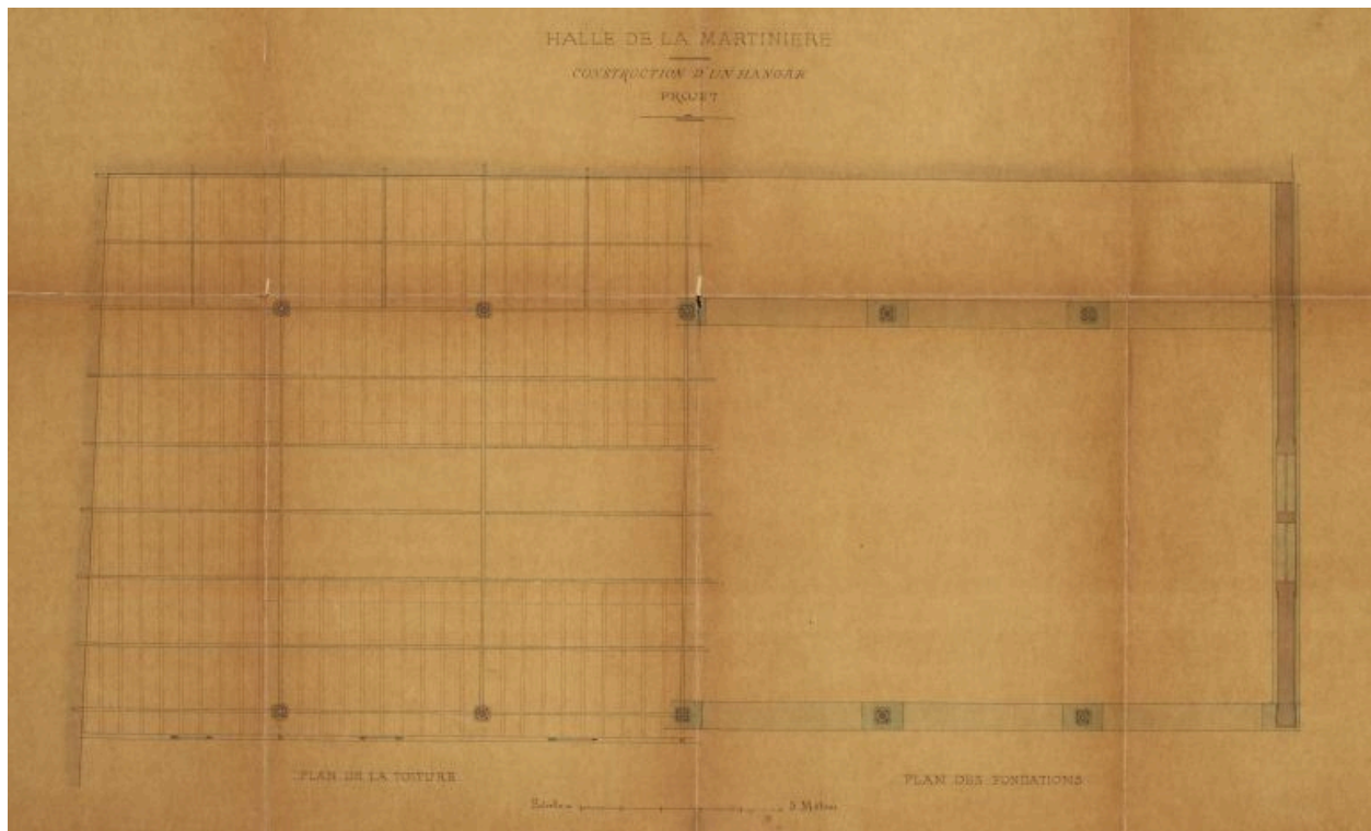
Halle de la Martinière, construction d'un hangar, plan des fondations et plan de la toiture
