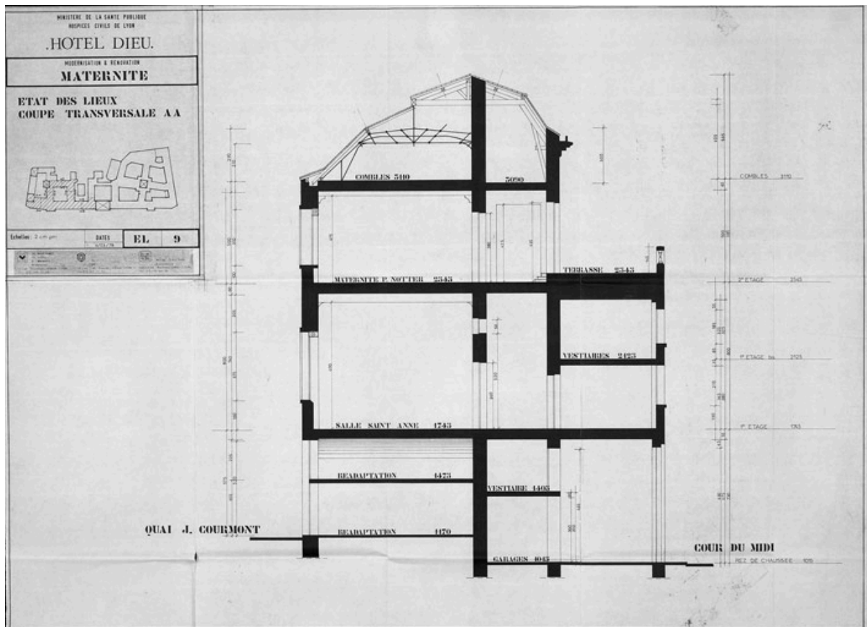
Modernisation et rénovation, maternité. Etat des lieux. Mortamet/Vidal/Manhes. SLETTI. BETSE Caillaud. Coupe transversale AA, 6 mars 1978
