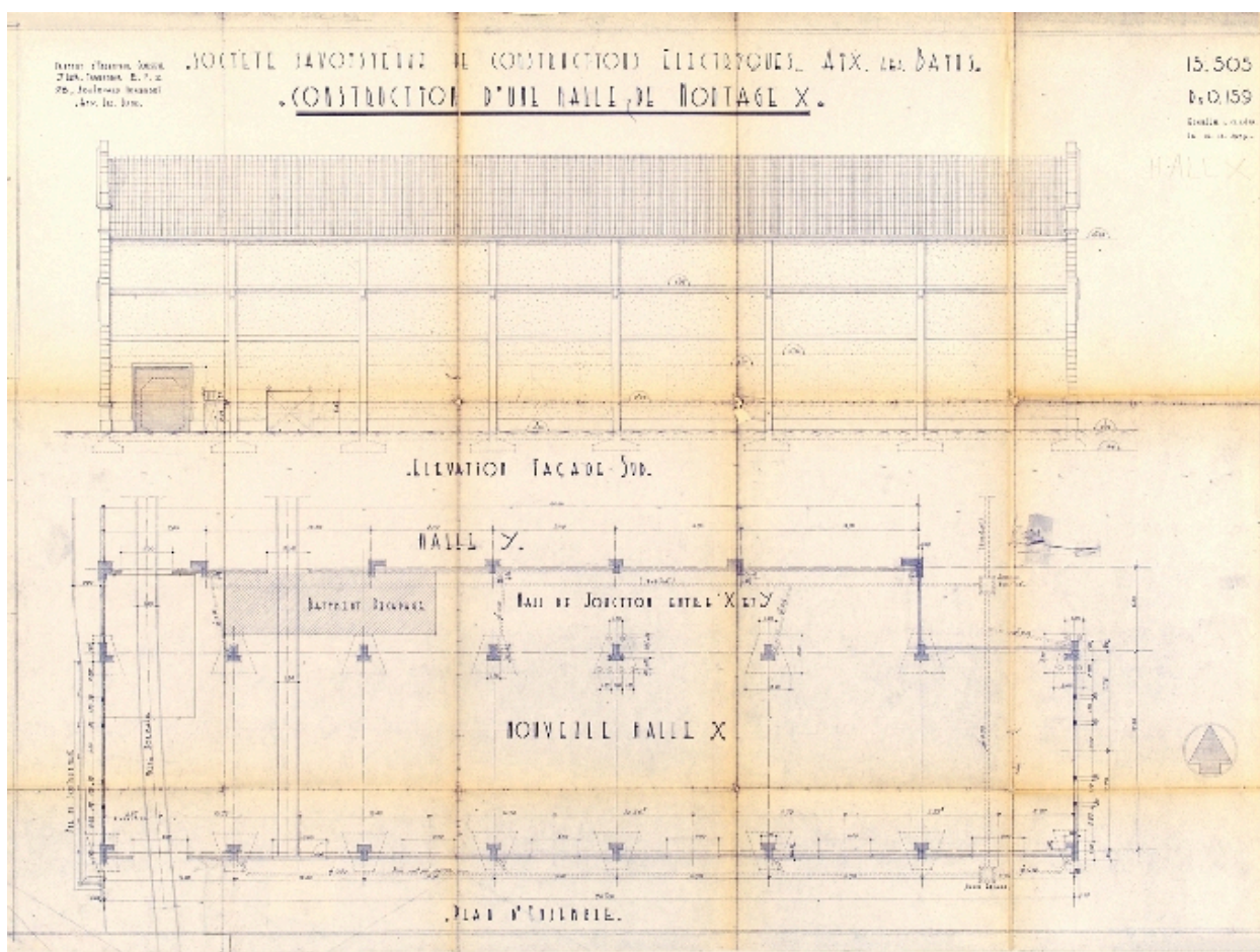
Plan et élévation sud de la halle X
