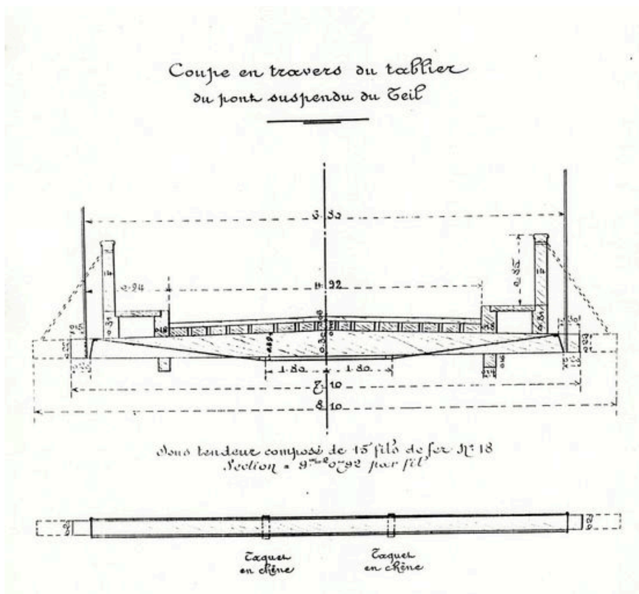
Coupe en travers du tablier du pont suspendu du Teil, l'ingénieur ordinaire, 4 décembre 1911 (AD Ardèche, 2S30/11)
