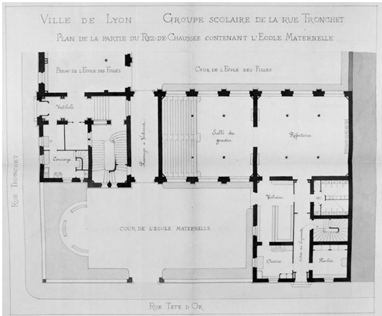
Plan de la partie du rez-de-chaussée contenant l'école maternelle
