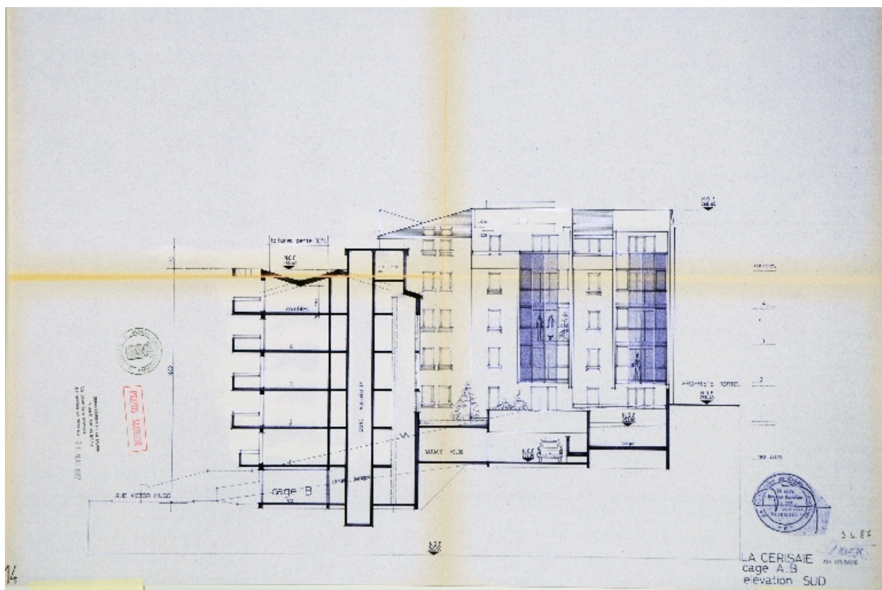
Élévation sud
