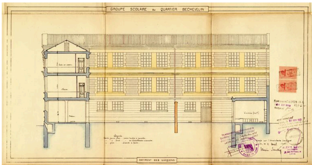
Bâtiment des garçons, élévation nord, 1921. Dessin à la plume ( AC Lyon. 0476 WP 54)
