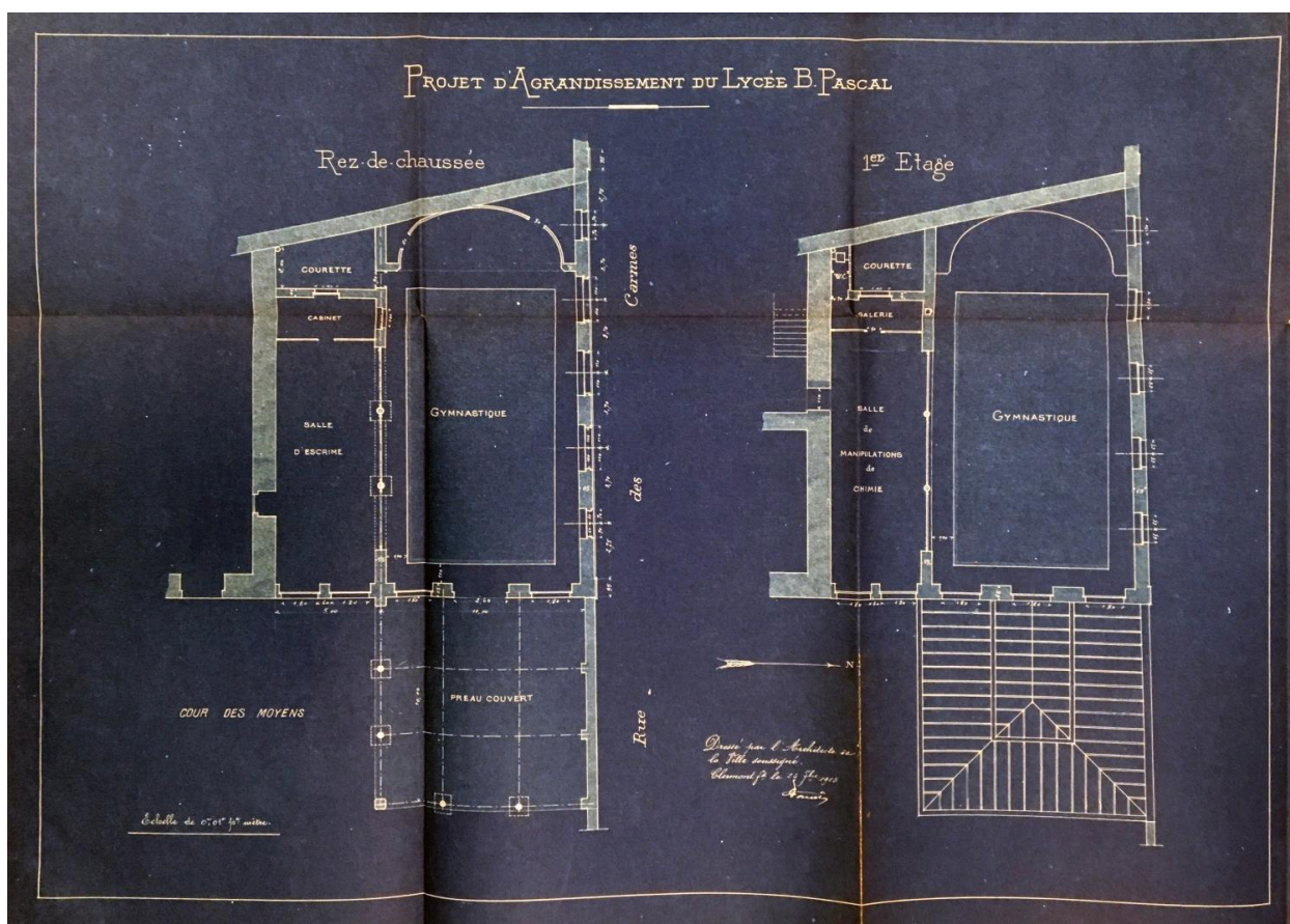
Projet d'agrandissement par Poncelet, 1905 : plans du rez-de-chaussée et du 1er étage (AC Clermont-Ferrand, 4 M 1/13)
