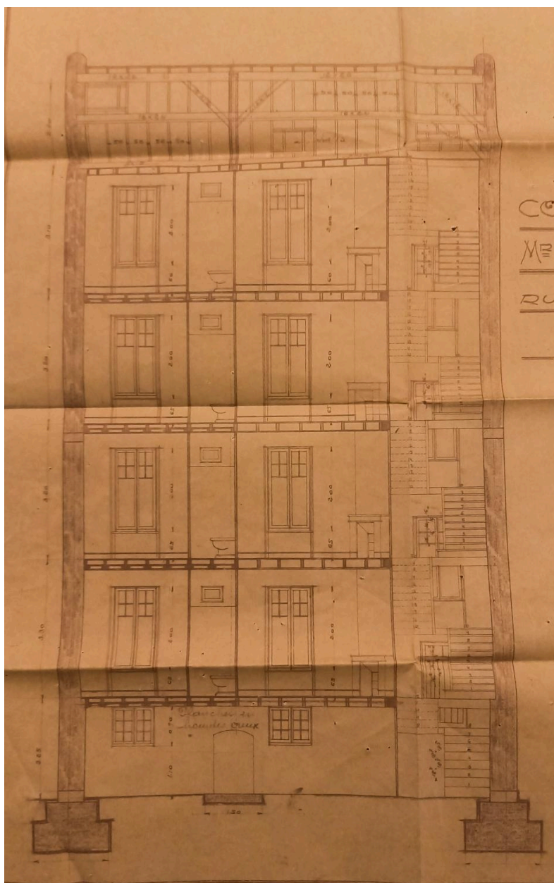
Coupe transversale. 25 rue Antoine-Raynaud. Edifice de comparaison
