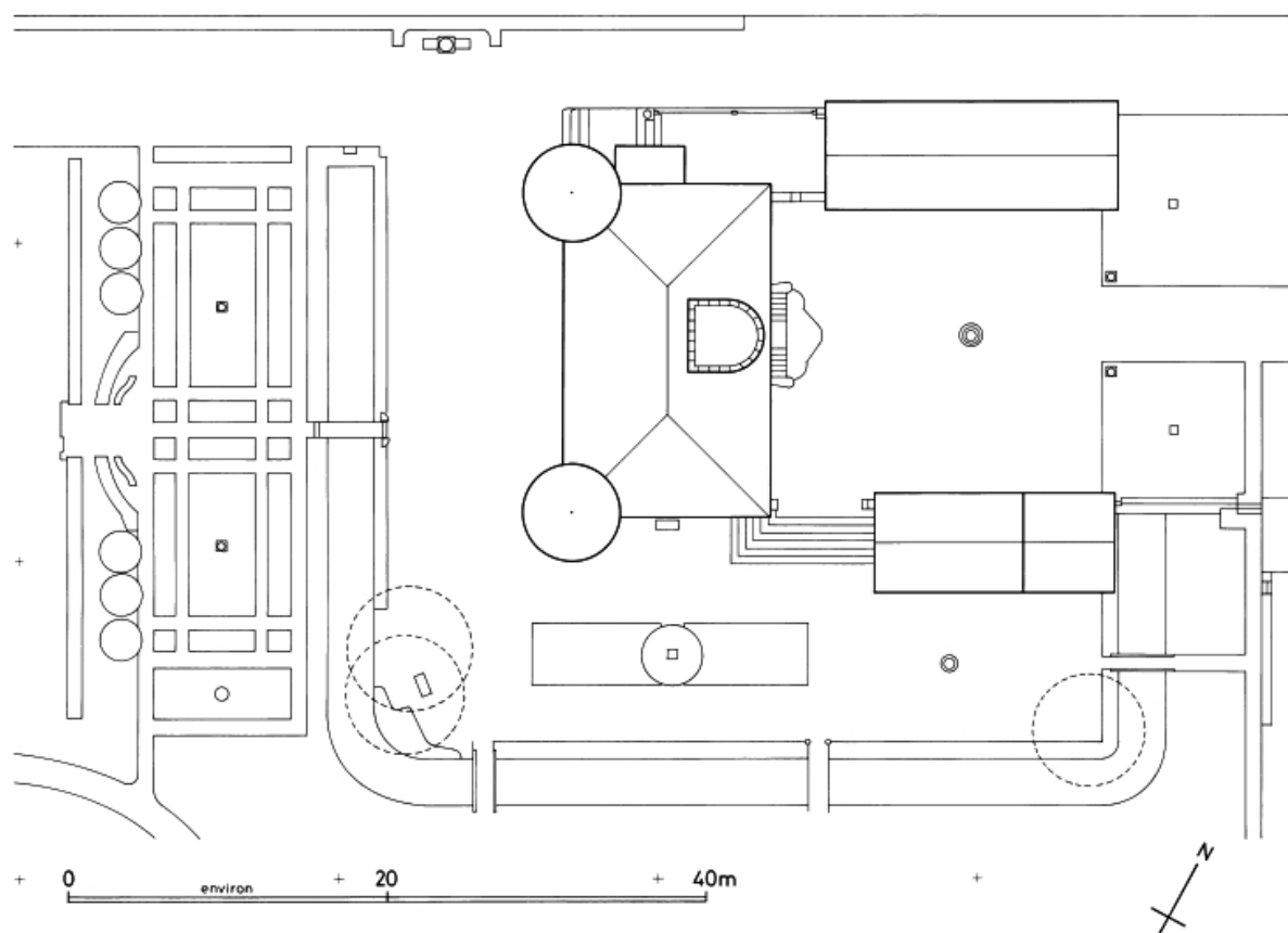
Plan masse et de toiture. Relevé schématique.
