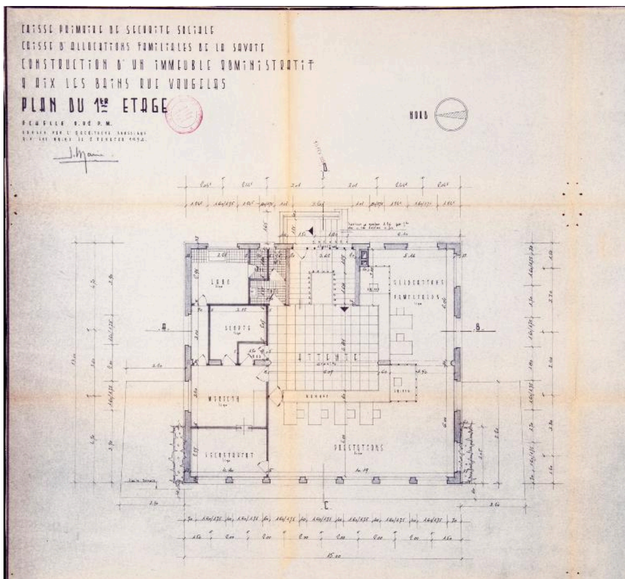
Plan du 1er étage, 1954
