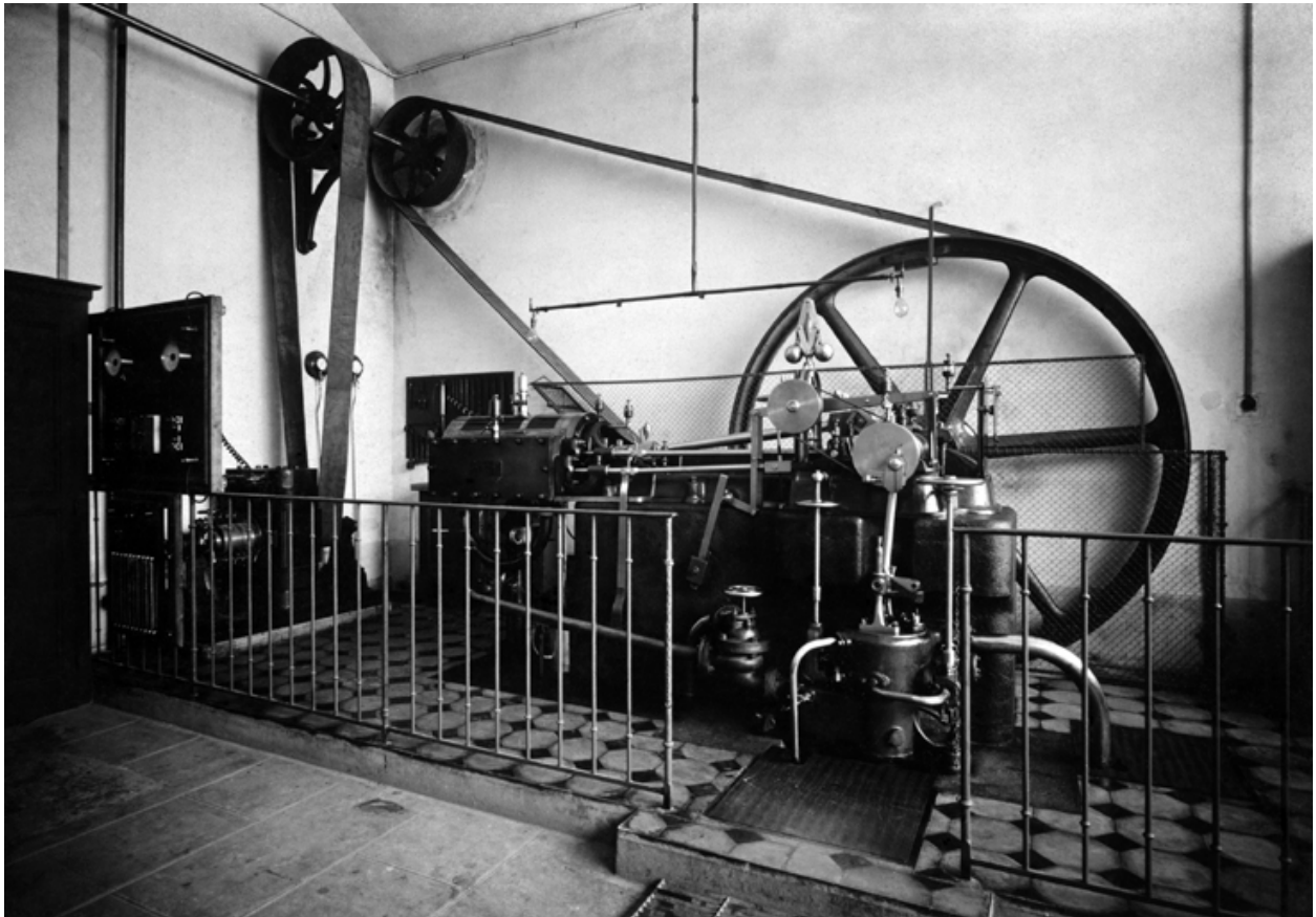
Vers 1895, station électrique.
