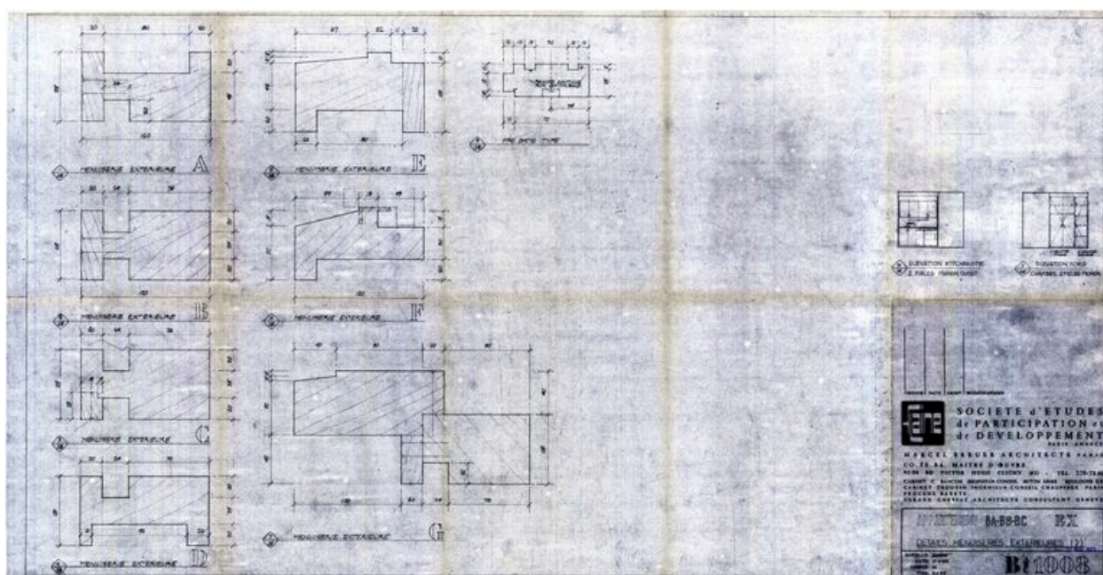
Détails des menuiseries extérieures (2). Marcel Breuer architecte, 27 novembre 1972 (AC Magland)
