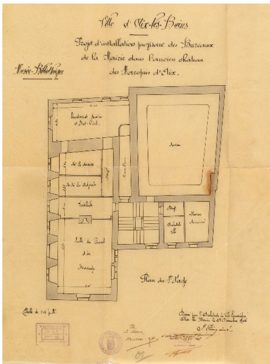
Plan du 1er étage
