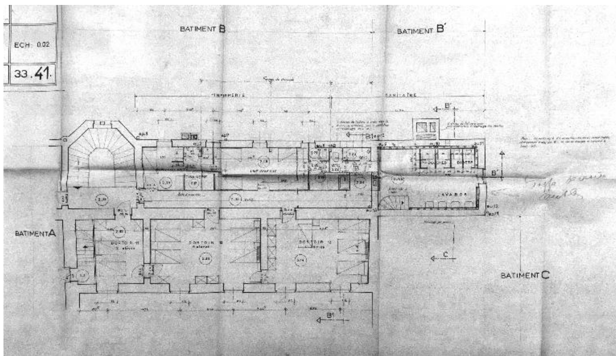
Château, corps de bâtiment BB' : plan d'exécution, 2e étage, 1955 (AD Loire, 690 VT 39)
