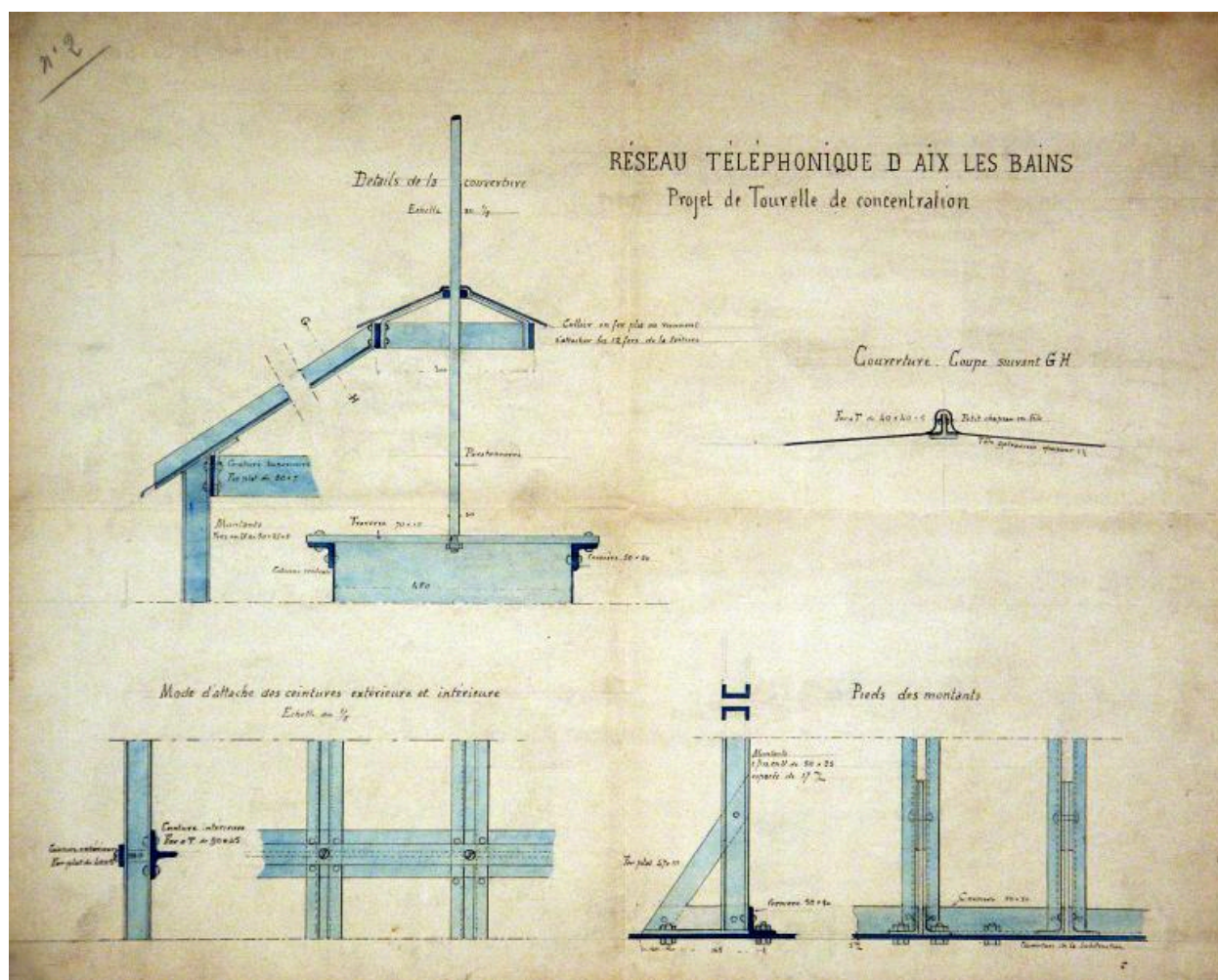
Projet de tourelle de concentration, 1907
